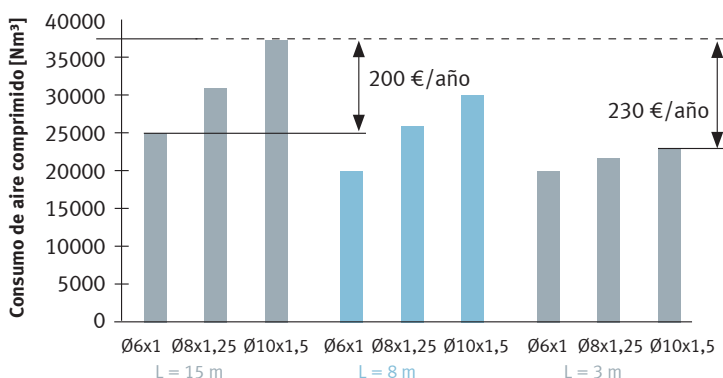
Consumo anual de aire comprimido [Nm 3 ] de 10 cilindros de sujeción, 1500 ciclos/día
